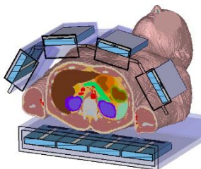
2 Spulenmodell mit anatomischem Körpermodell
